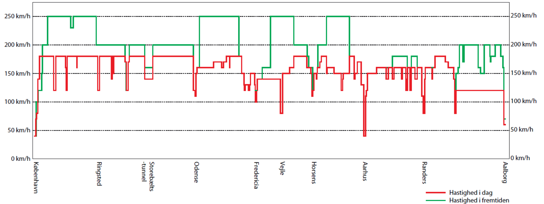
Figur 59. Hastigheder idag og i fremtiden - højere hastighed på hele banen mellem København og Aalborg
