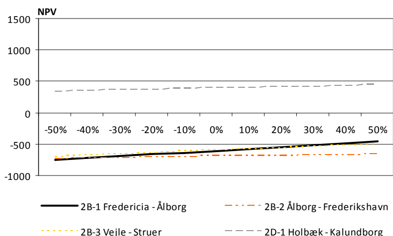
Figur 16: Betydningen for nutidsværdien af ændringer i både el- og dieselpris, fortsættelsesscenarier
